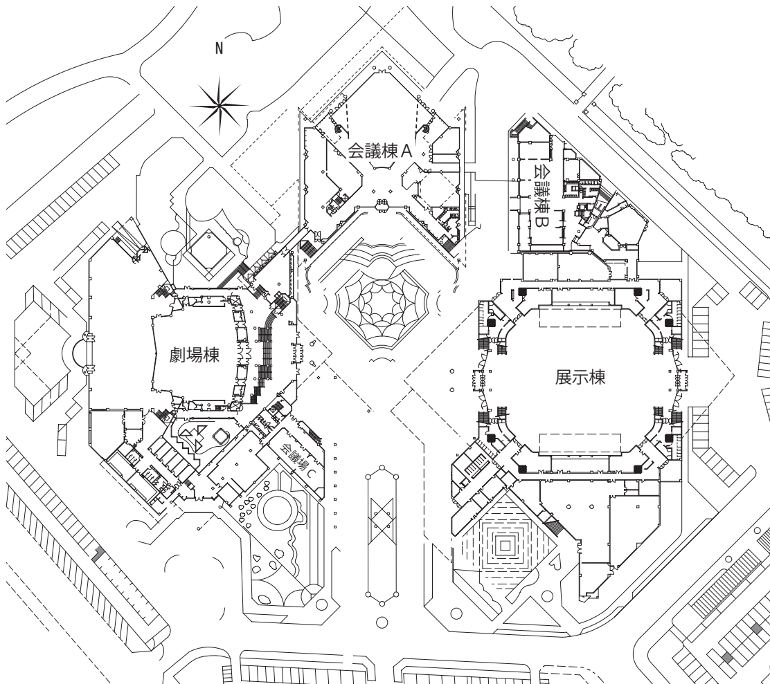
全体配置図
